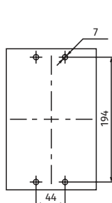
Размеры установки на щите 3 полюса
