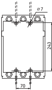
Размеры установки на щите 3 полюса
