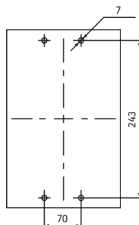
Размеры установки на щите 3 полюса
