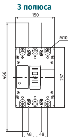
Размеры установки на щите 3 полюса
