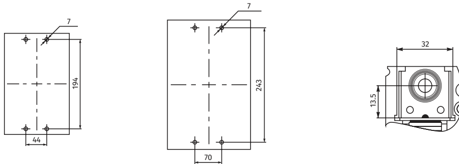
Размеры установки на щите
