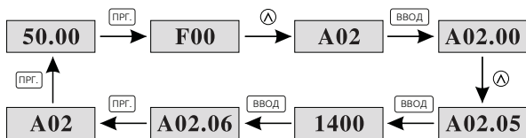
Рисунок 4-5. Отображение скорости вращения.
